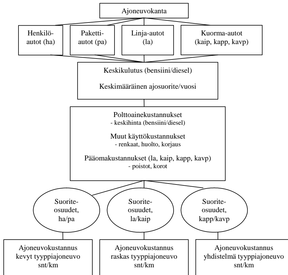
Kuva 1. Ajoneuvokustannusten muodostaminen.
